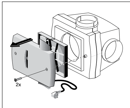
Fig. 9 Openen voorkap
