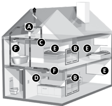
Fig. 1 Overzicht ventilatiesysteem Compact-10RH
