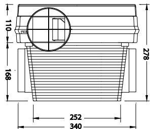
Fig. 3 Bovenaanzicht
