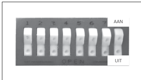
Fig. 8 Dipswitch schakelaars op UIT in Compact-10RH
