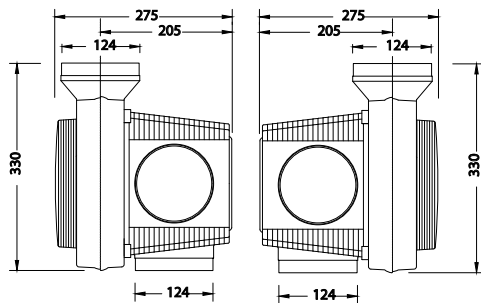
Fig. 2 Zijaanzichten
