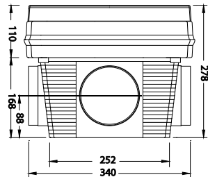
Fig. 5 Onderaanzicht
