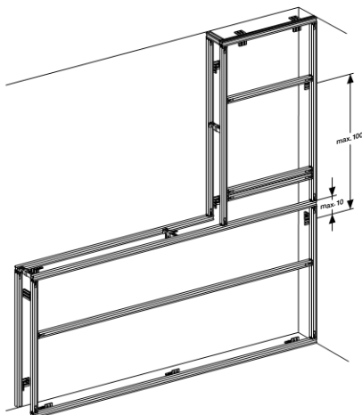
Afbeelding 226: GIS voorwand met horizontale overgangen
