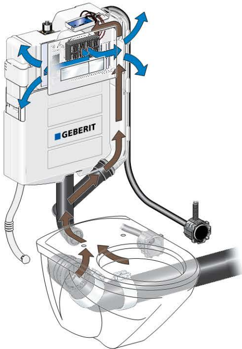
Afbeelding 214: Geurafzuiging circulatielucht
