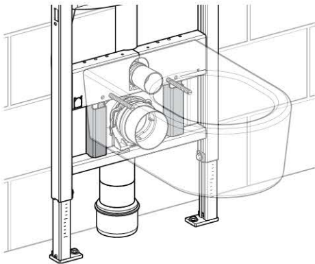
Afbeelding 216: Steun voor WC-keramiek met klein contactvlak aan hand van het voorbeeld Geberit Duofix
