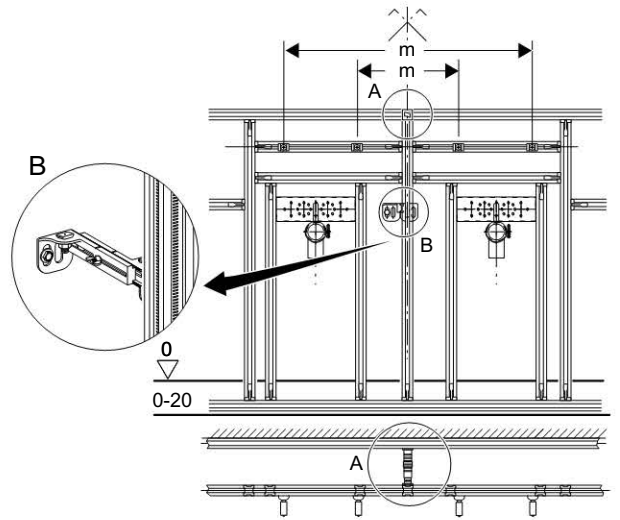
Afbeelding 222: Dubbele wastafel met maximaal 5 bevestigingen, 2 aansluitingen
