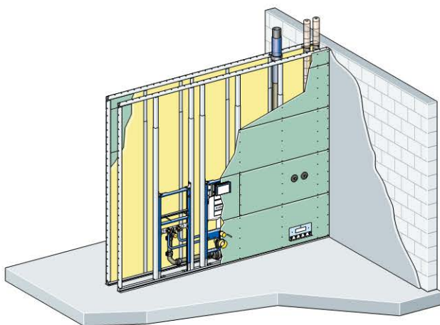
Afbeelding 179: Duofix systeem scheidingwand installatie
