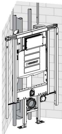
Inbouw in de hoek met val- en standleidingen
