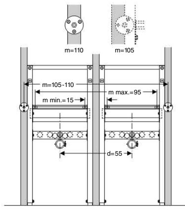
Afbeelding 192: Dubbele wastafel met asafstand 55 cm / 3 systeem standers of deelhoge standers
