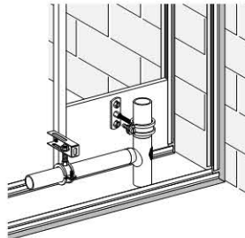
Afbeelding 197: Leidingsbevestiging aan de Duofix draagconstructie
