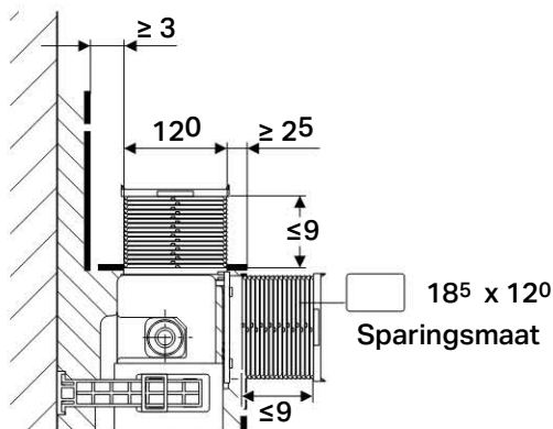
Afbeelding 239: Afwerklaagdikte voor bedieningsplaten Omega20, Omega30 en Omega60
