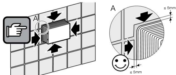
Afbeelding 241: Maximale afstand van de springkoker tot de betegelde wand
