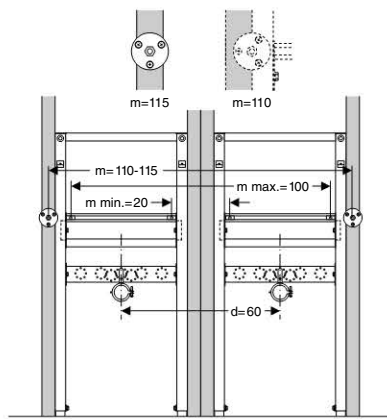
Afbeelding 193: Dubbele wastafel met asafstand 60 cm / 4 systeem standers of deelhoge standers
