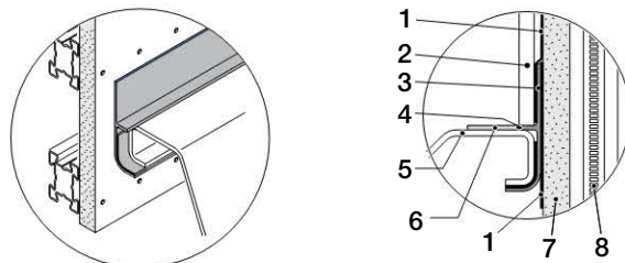
Afbeelding 175: Kuip-/bakafdichting en ont koppeling met Geberit voegband
