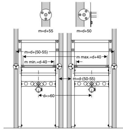
Afbeelding 194: Dubbele wastafel met asafstand > 60 cm / 4 systeem standers of deelhoge standers
