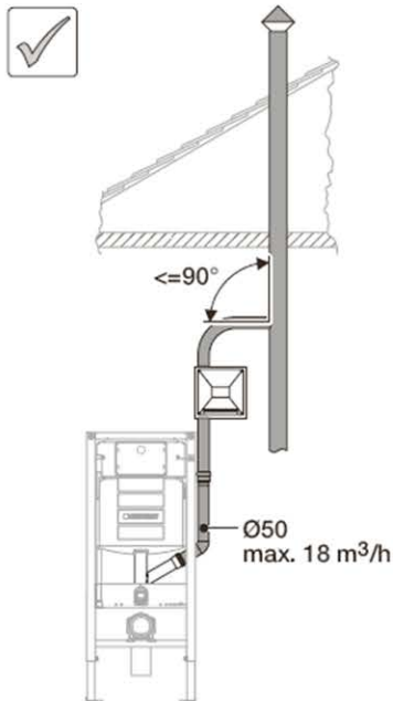
Afbeelding 170: Aansluiting van de wand-WC aan een secundaire ontlufting
